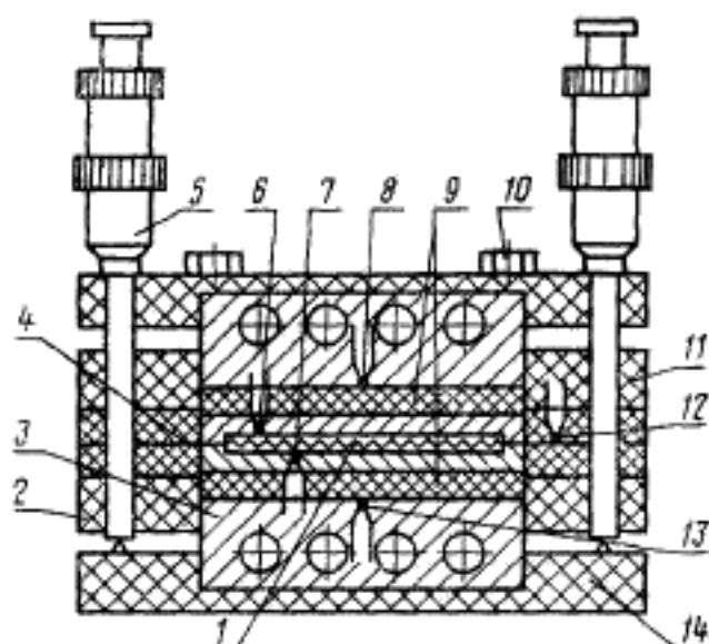
1—нагреватель; 2, 11—текстолитовые кольца; 3—холодильники; 4—тепломер; 5—микрометры; 6, 7, 8, 12, 13—термомпары; 9—образцы; 10—прижимные винты; 14—текстолитовые крышки
