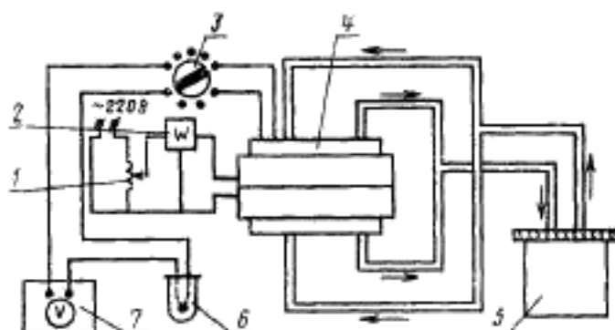
1—автотрансформатор; 2—ваттметр; 3—переключатель термомонитор; 4—рабочая часть; 5—термостат; 6—холодный спай термомпар; 7—электронно-цифровой вольтметр
