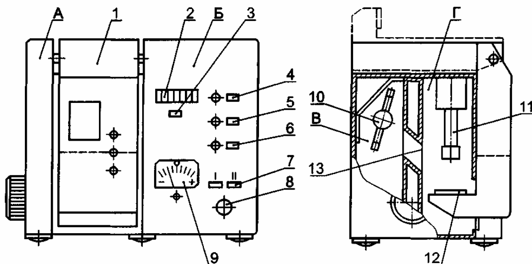
A — блок индексации; B — электронный блок управления; B — отсек излучателя; Г — испытательный отсек; 1 — кювета; 2 — счетчик времени; 3 — кнопка сброса счетчика времени; 4 — кнопка выключения прибора; 5 — кнопка выключения ртутной лампы; 6 — кнопка выключения ФЭУ; 7 — кнопка переключения режимов; 8 — индикатор напряжения; 9 — регулятор порога чувствительности; 10 — ртутная лампа ДРК 120; 11 — фотоэлектронный умножитель; 12 — кассета с образцом; 13 — светофильтр УФС-8
