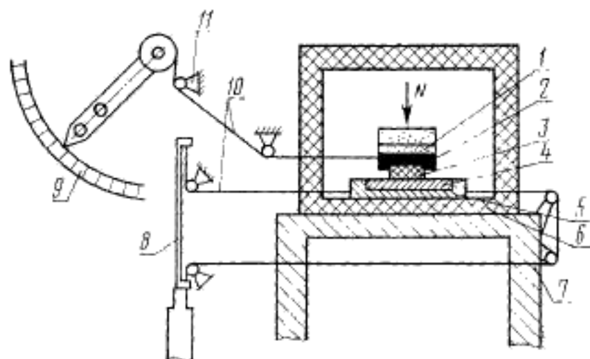
Установка по определению коэффициента трения
