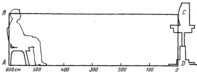
Схема расположения испытателя и прибора типа ПОЗД-2
