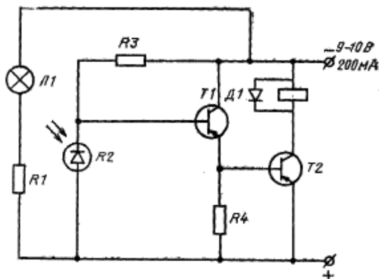
Электрическая схема автоматического датчика
