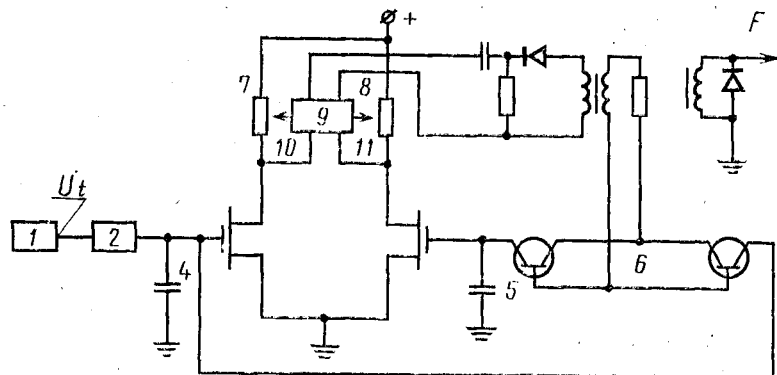
Принципиальная электрическая схема устройства для измерения скорости изменения температур
