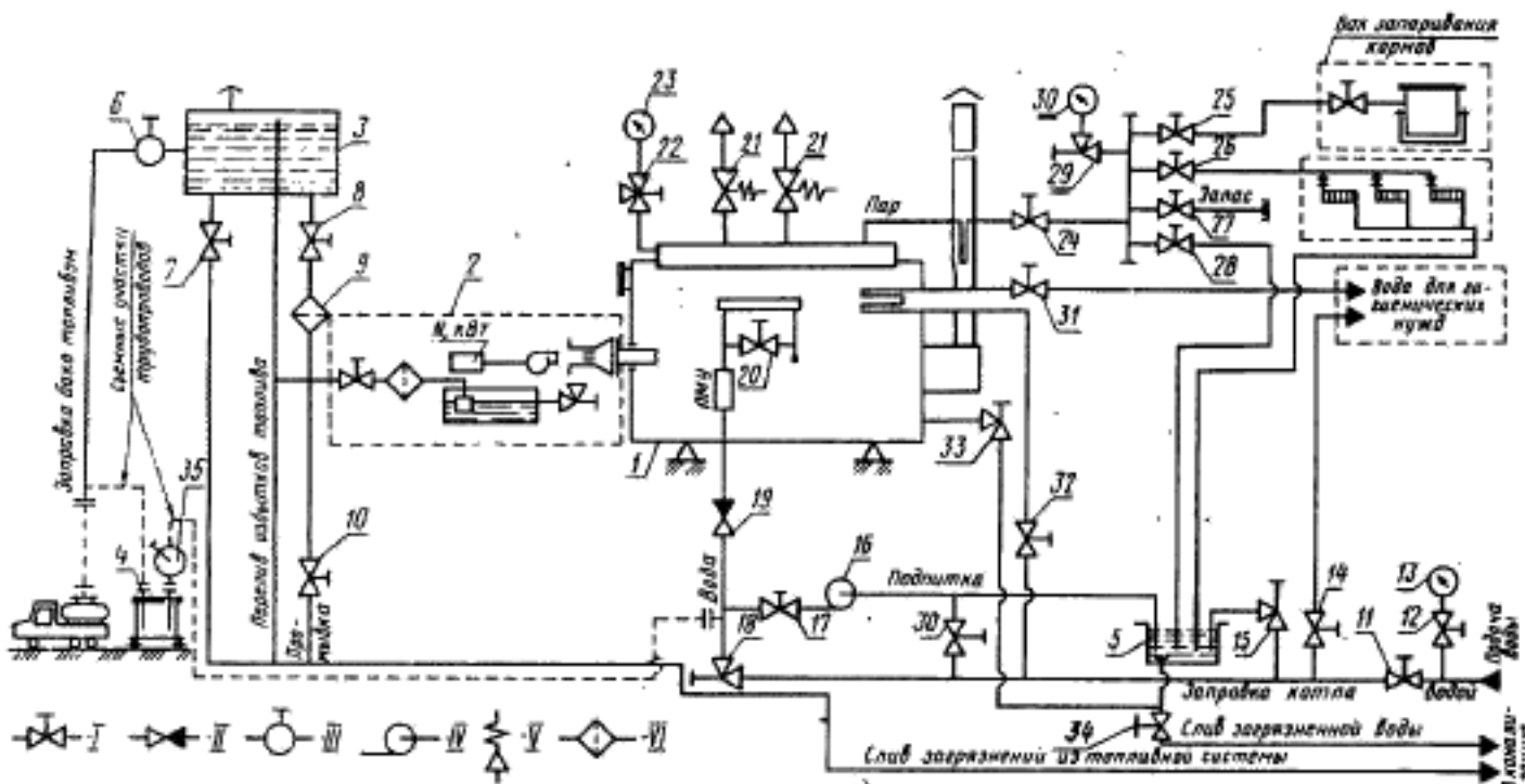
Схема котла КВ-300 М в сборе
