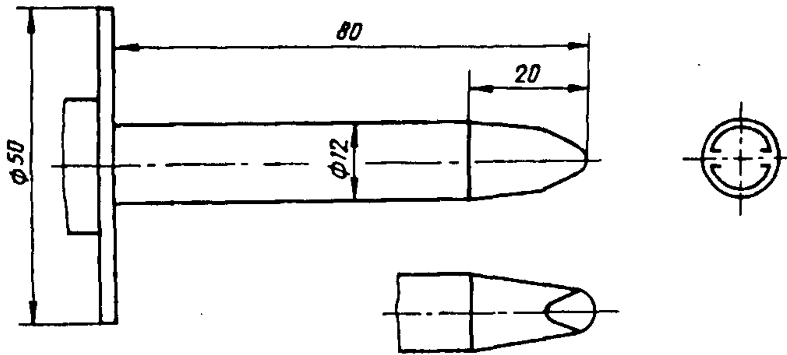
Размеры, мм, наконечника пальца — по рисунку 1а
