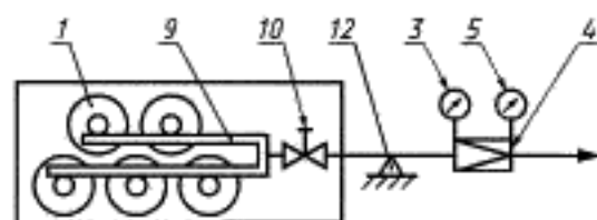
г) Рампа с баллонами, соединенными в группу
