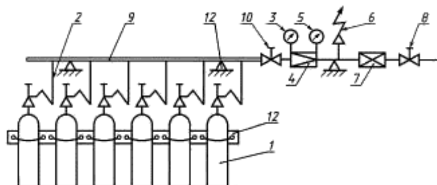
в) Рампа с более 6 баллонами
