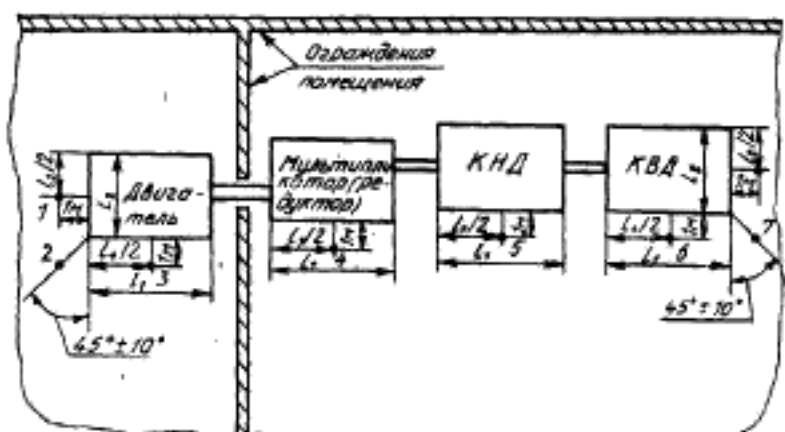
1—7 — точки измерения шума; КНД — корпус низкого давления компрессора; КВД — корпус высокого давления компрессора; l_1 и l_2 — длины и ширина обтекающего источника шума параллелепипеда
