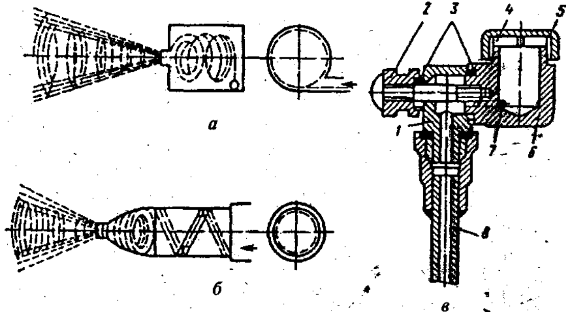
Рис. 14 Принцип действия (а, б) и устройство (в) форсунок 1 - корпус, 2 - винт, 3 - прокладки, 4 - шайба, 5 - накидная гайка, 6 - рабочая головка, 7 - входное отверстие, 8 - канал
